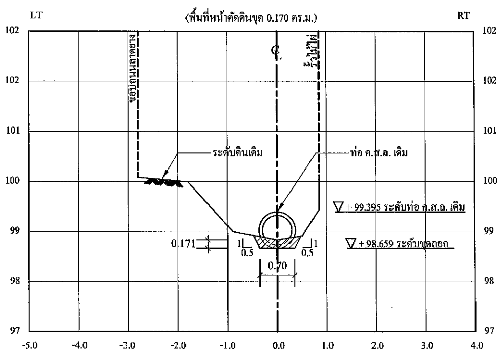
รูปตัดตามขวาง STA. 0+000
