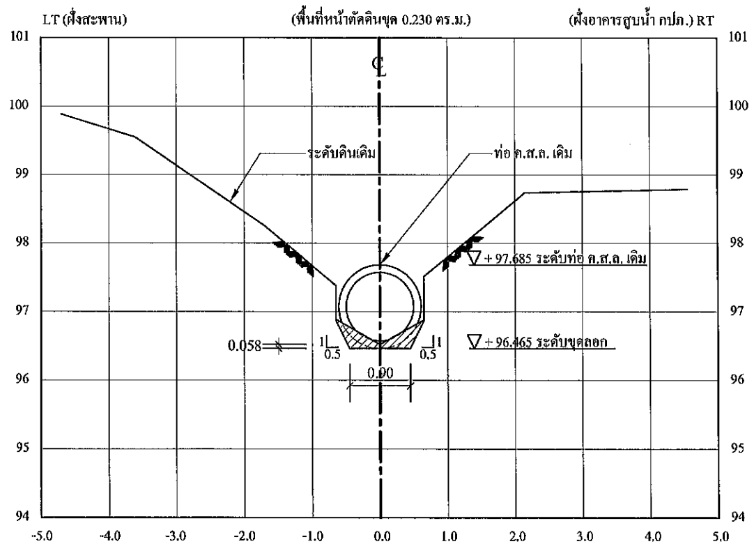
รูปตัดตามขวาง STA. 0+110.6
