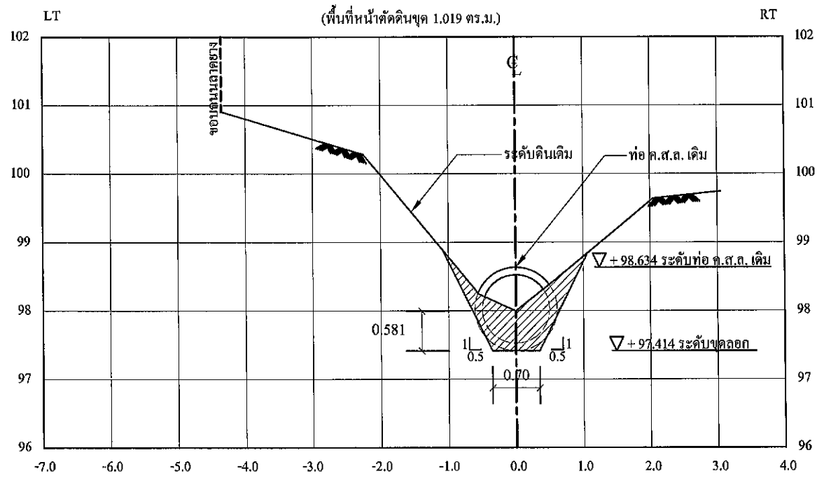
รูปตัดตามขวาง STA. 0+103.3
