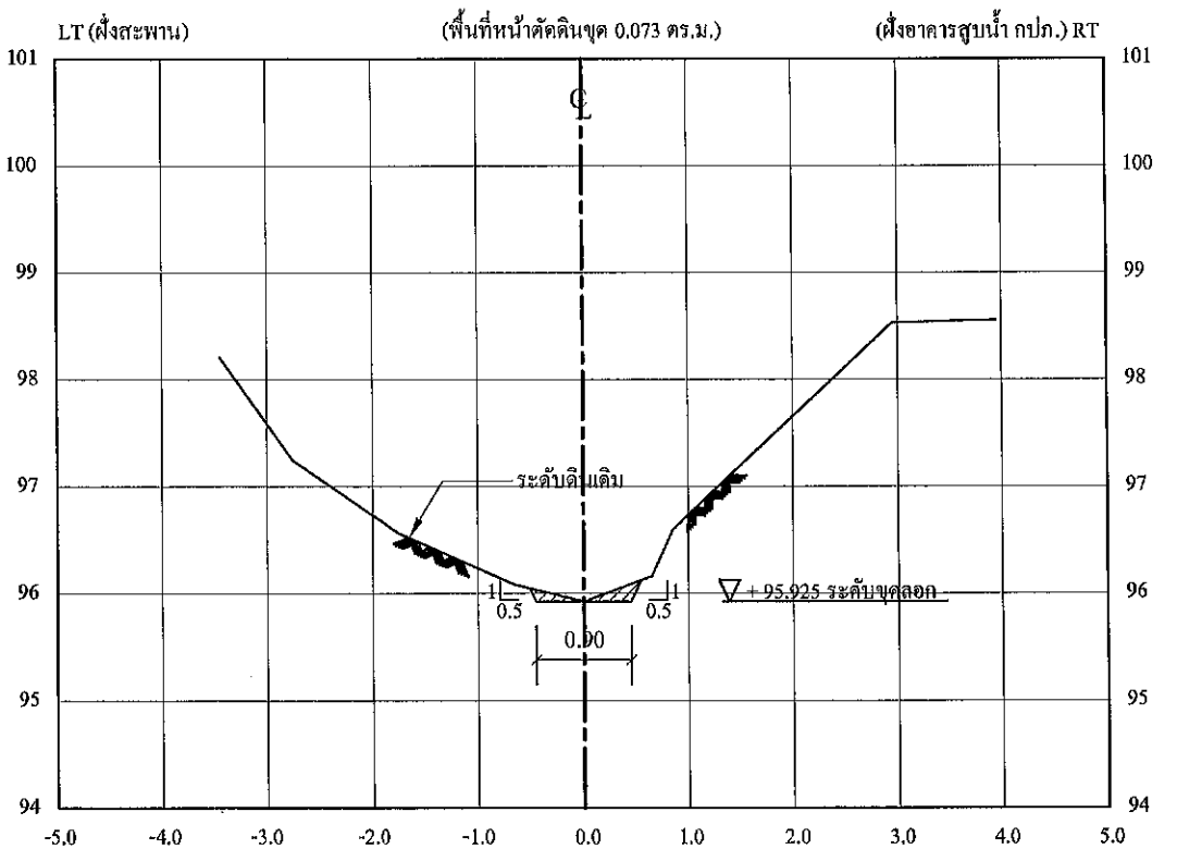
รูปตัดตามขวาง STA. 0+120
