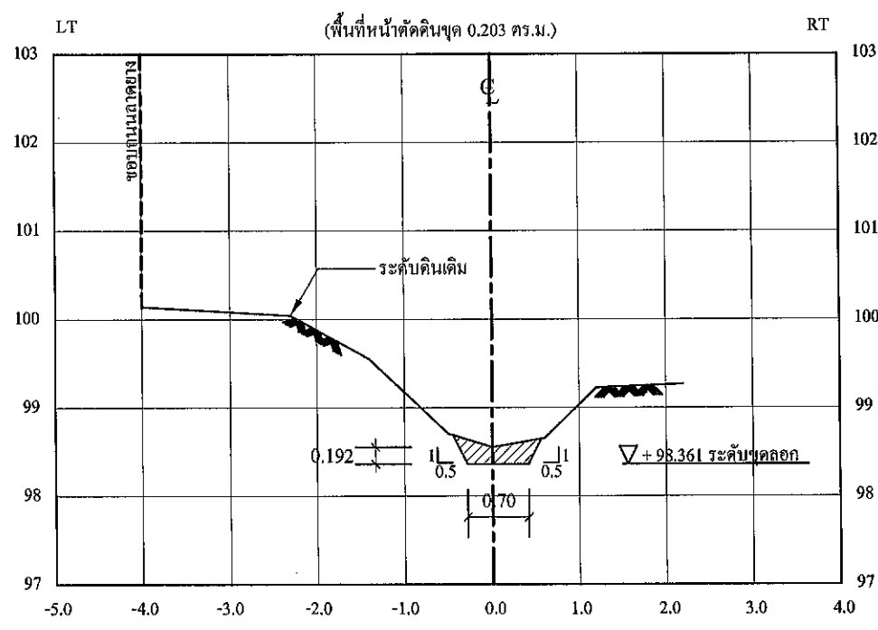
รูปตัดตามขวาง STA. 0+025
