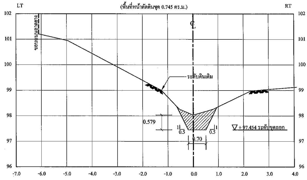
รูปตัดตามขวาง STA. 0+100
