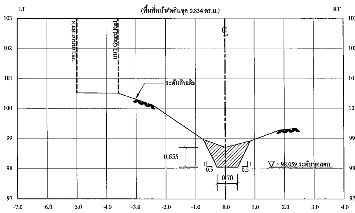
รูปตัดตามขวาง STA. 0+050
