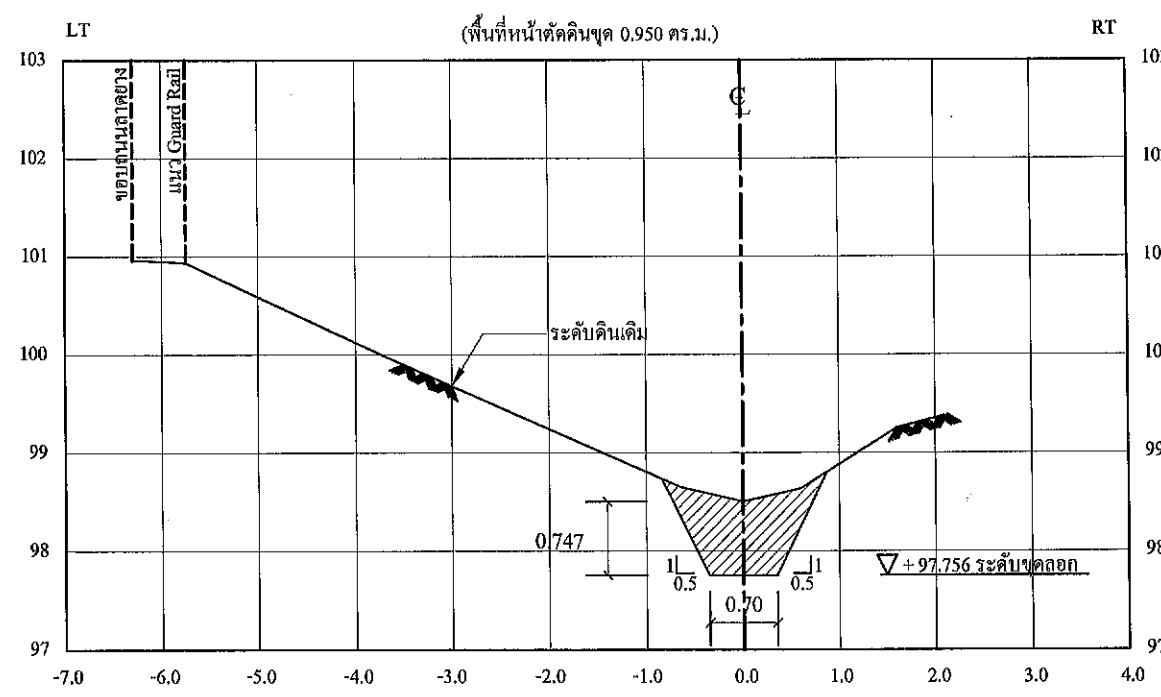
รูปตัดตามขวาง STA. 0+075
