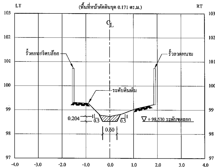
รูปตัดตามขวาง STA. 0+050
