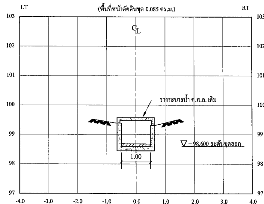
รูปตัดตามขวาง STA. 0+091.6
