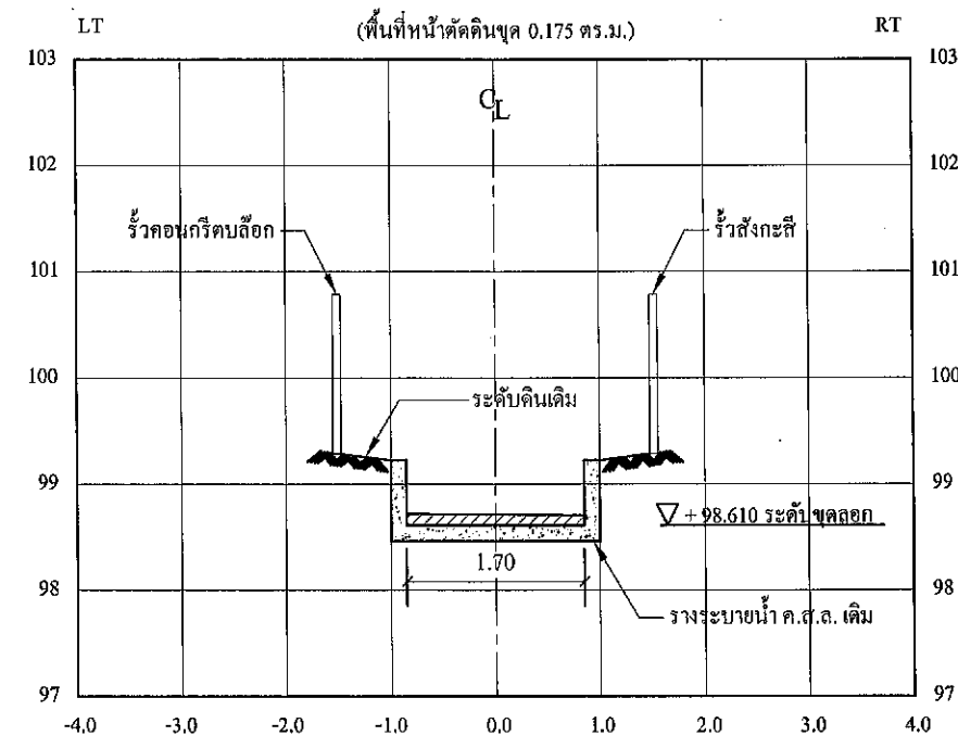
รูปตัดตามขวาง STA. 0+088.5
