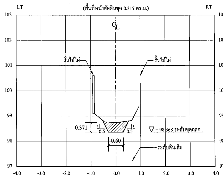
รูปตัดตามขวาง STA. 0+110
