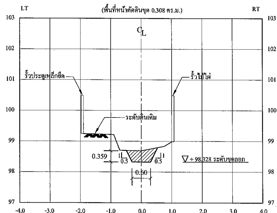
รูปตัดตามขวาง STA. 0+125
