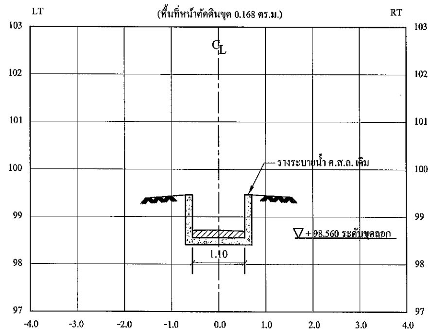
รูปตัดตามขวาง STA. 0+109.1
