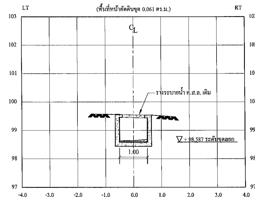
รูปตัดตามขวาง STA. 0+098.6
