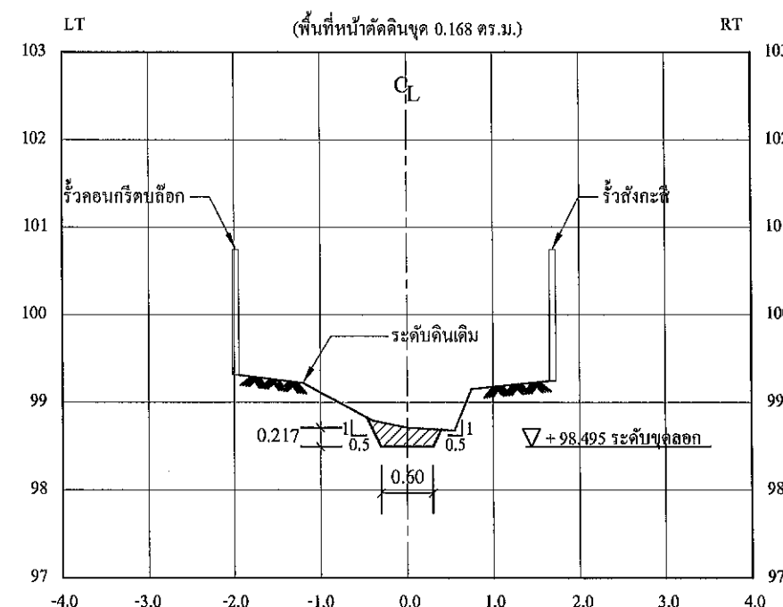
รูปตัดตามขวาง STA. 0+075
