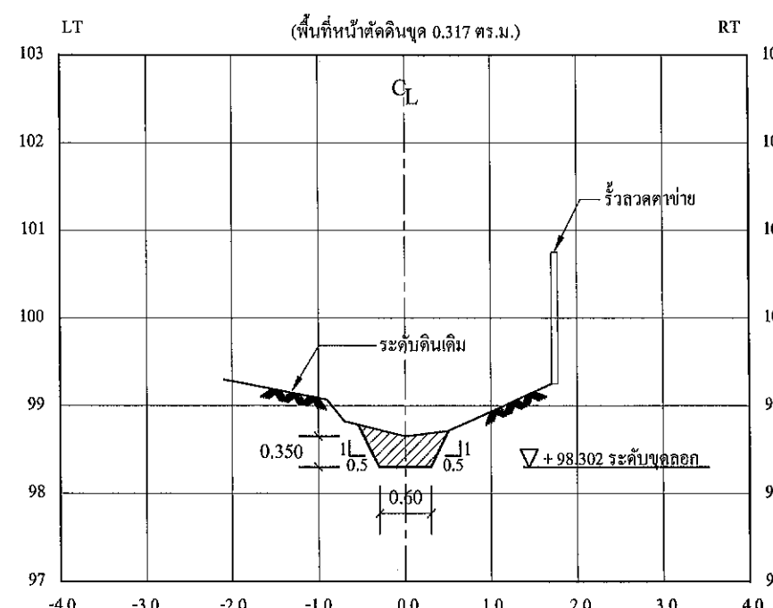
รูปตัดตามขวาง STA. 0+135
