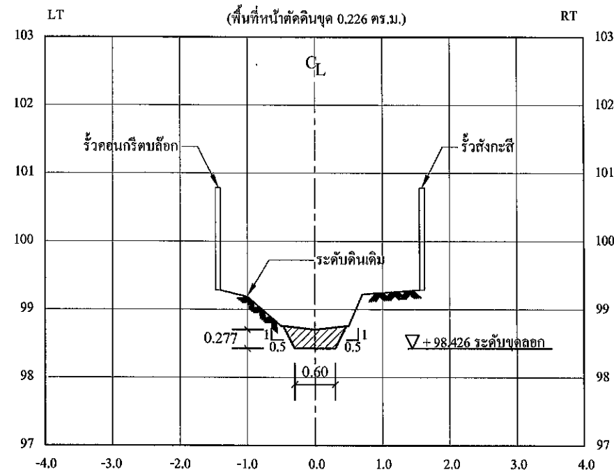
รูปตัดตามขวาง STA. 0+088
