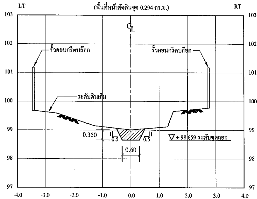
รูปตัดตามขวาง STA. 0+000
