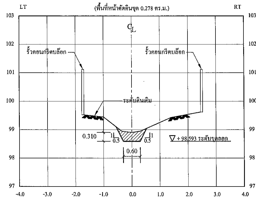
รูปตัดตามขวาง STA. 0+025
